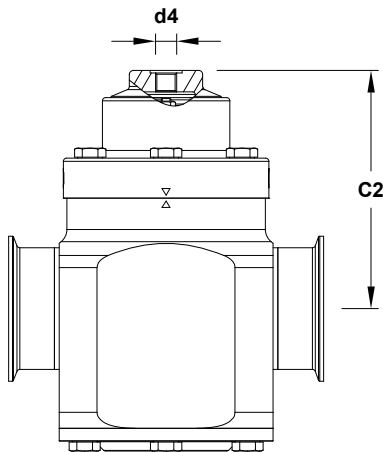
Optional dome-loading
