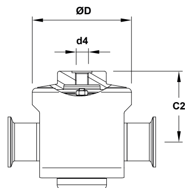
Optional dome-loading
